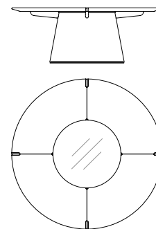
67010 Tavolo rotondo in noce canaletto inserto girevole in vetro glacé Round table in walnut canaletto lazy Susan in glacé glass cm Ø 200 x h 75 in Ø 78 3/4 x h 29 1/2
